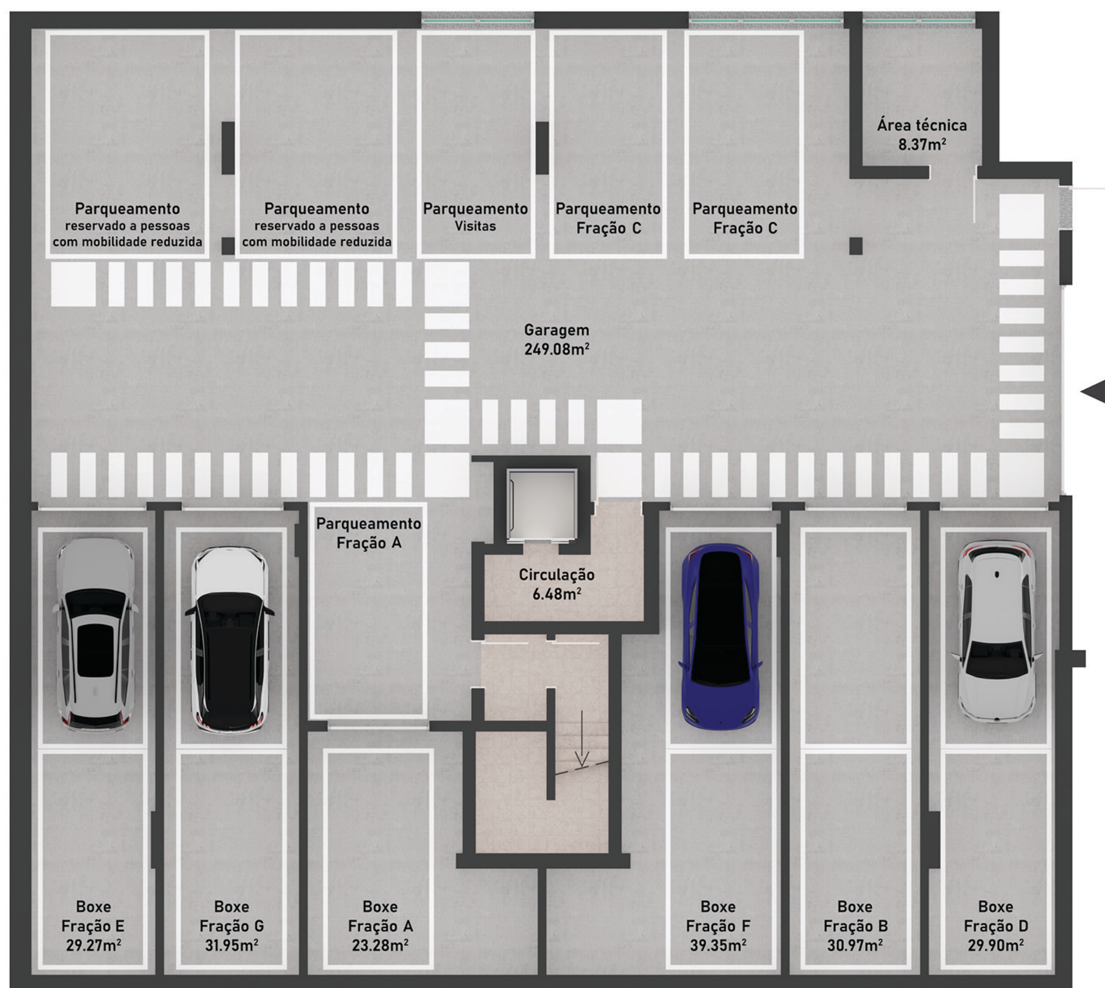
Piso -2
