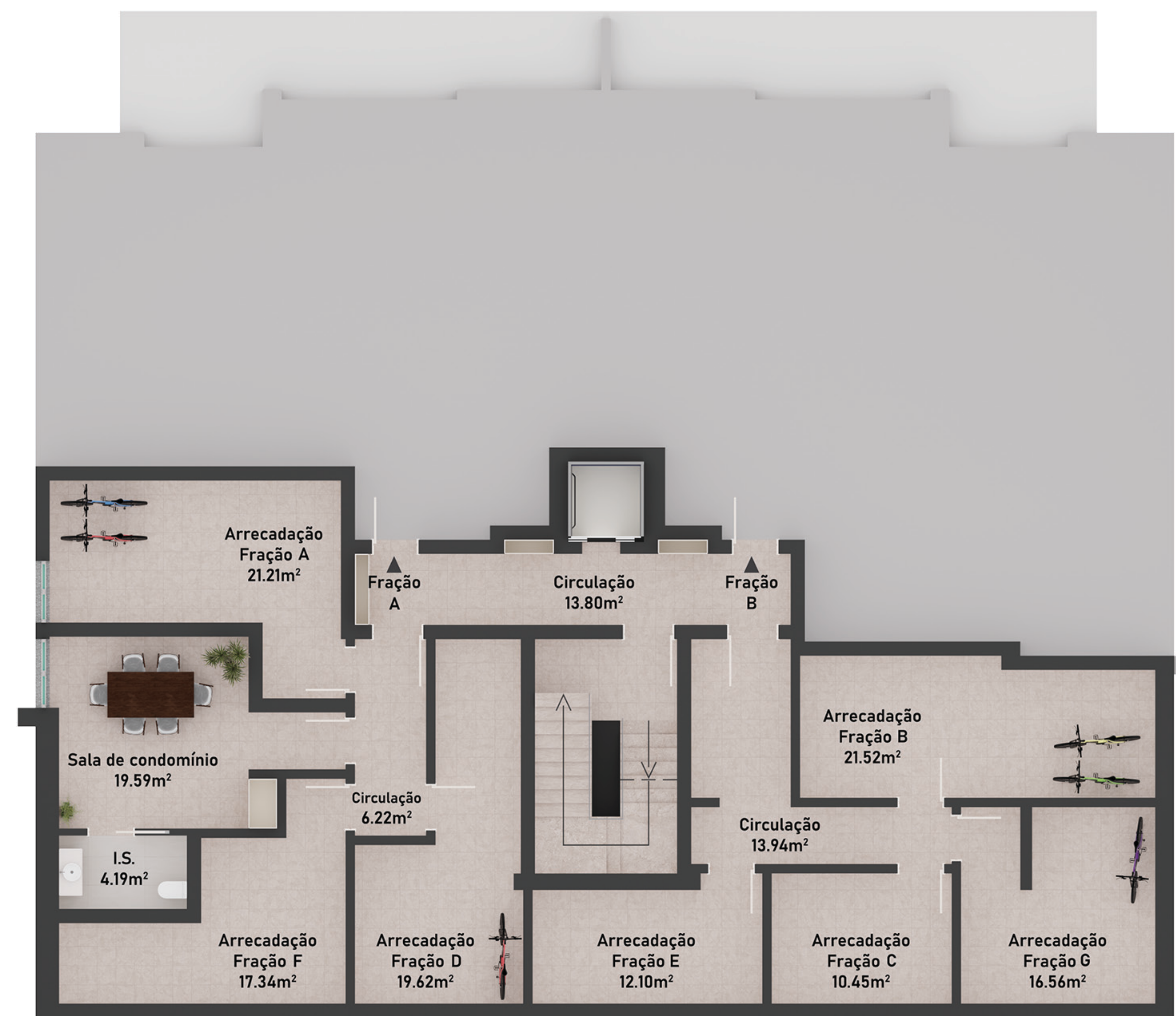
Piso -1
